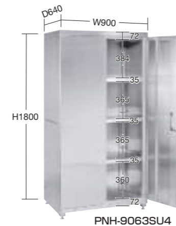
PNH-9063SU4
