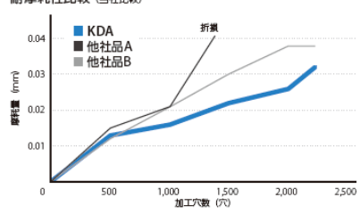
耐摩耗性比較 (当社比較)
