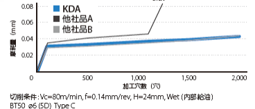
ステンレス鋼 SUS304 (当社比較)
