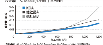
合金鋼 SCM440 (32HRC) (当社比較)
