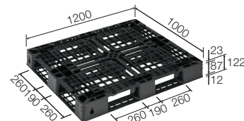
パレット D4-1012-13
