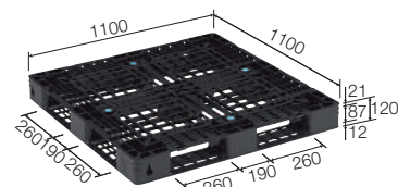
パレット D4-1111-11
