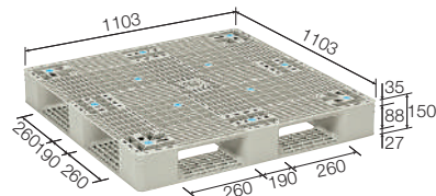
パレット GT-1111D4
