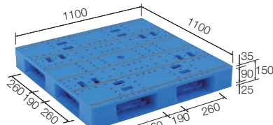
パレット LX-1111D4
