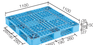
パレット D4-1111-6N
