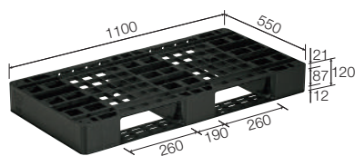
パレット D2-055110
